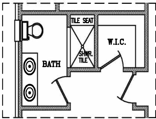
OPTIONAL DELUXE BATH
